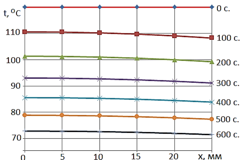
Рис. 3. Эпюра температуры по толщине пластины для разных значений времени
