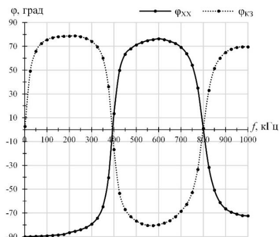
Рис. 2. ФЧХ характеристики Z_{BX} в режимах ХХ и КЗ линии.
