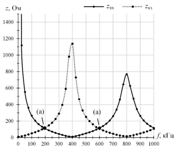
Рис. 1. АЧХ характеристики Z_{BX} в режимах ХХ и КЗ линии.
