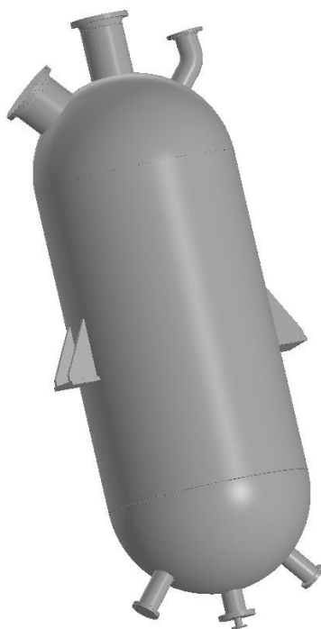
Параметрическая моделирование реактора каталитического риформинга в «Компас-МАКРО»
