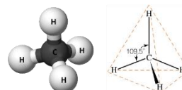
Рис. 1 Строение молекулы метана
