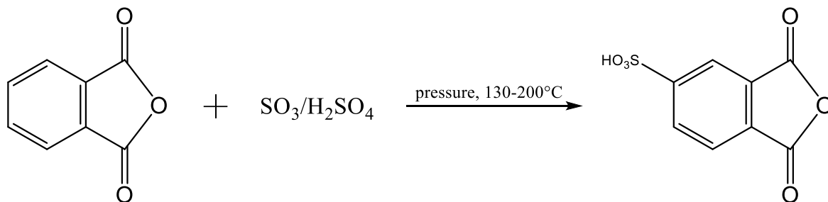
Рис. 2. Схема синтеза 4-сульфофталевого ангидрида
