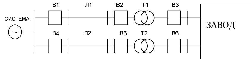
Рис. П 17. Схема электроснабжения завода.
