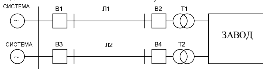
Рис. П 20. Схема электроснабжения завода.
