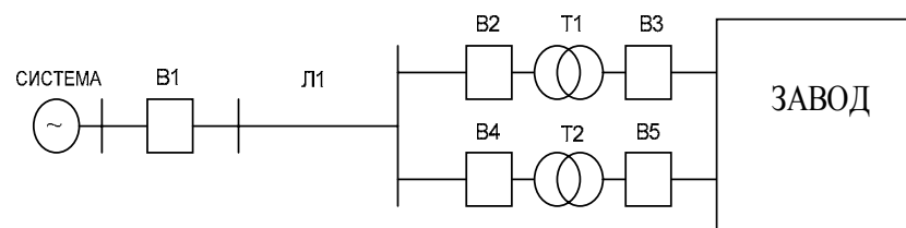
Рис. П 13. Схема электроснабжения завода.
