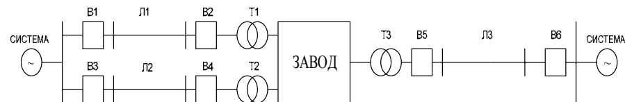
Рис. П 19. Схема электроснабжения завода.
