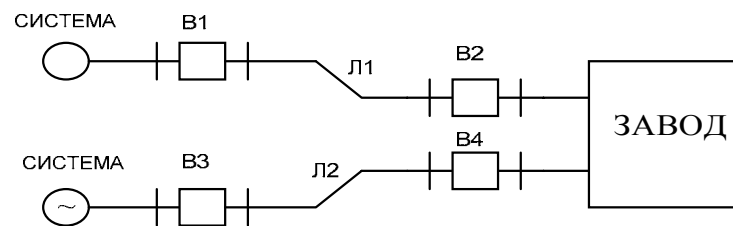
Рис. П 3. Схема электроснабжения завода.
