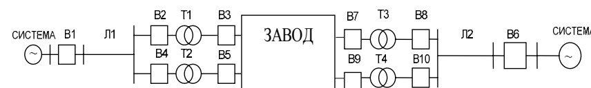
Рис. П 15. Схема электроснабжения завода.
