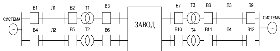
Рис. П 18. схема электроснабжения завода.
