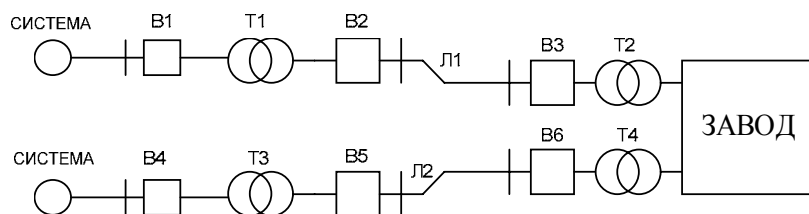
Рис. П 4. Схема электроснабжения завода.
