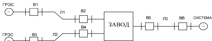
Рис. П 2. Схема электроснабжения завода.
