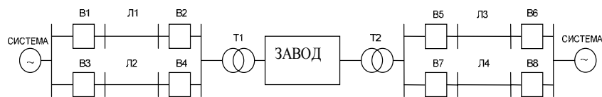
Рис. П 16. Схема электроснабжения завода.
