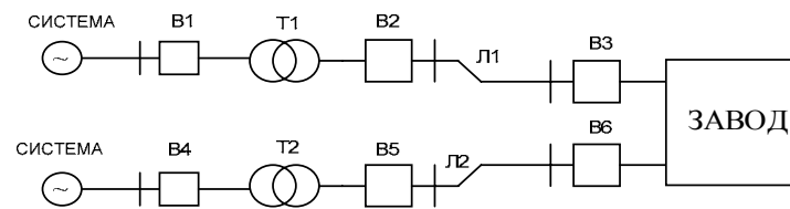
Рис. П 5. Схема электроснабжения завода.
