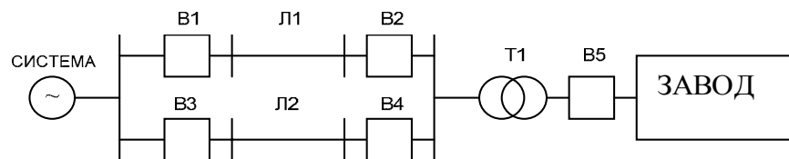
Рис. П 14. Схема электроснабжения завода.
