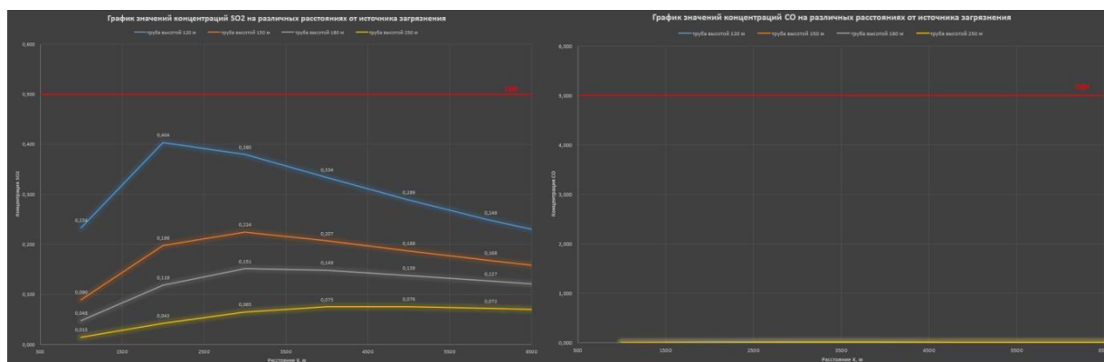
Рис. 2. Графики значений концентраций сернистого ангидрида (слева) и углерода оксида (справа)
