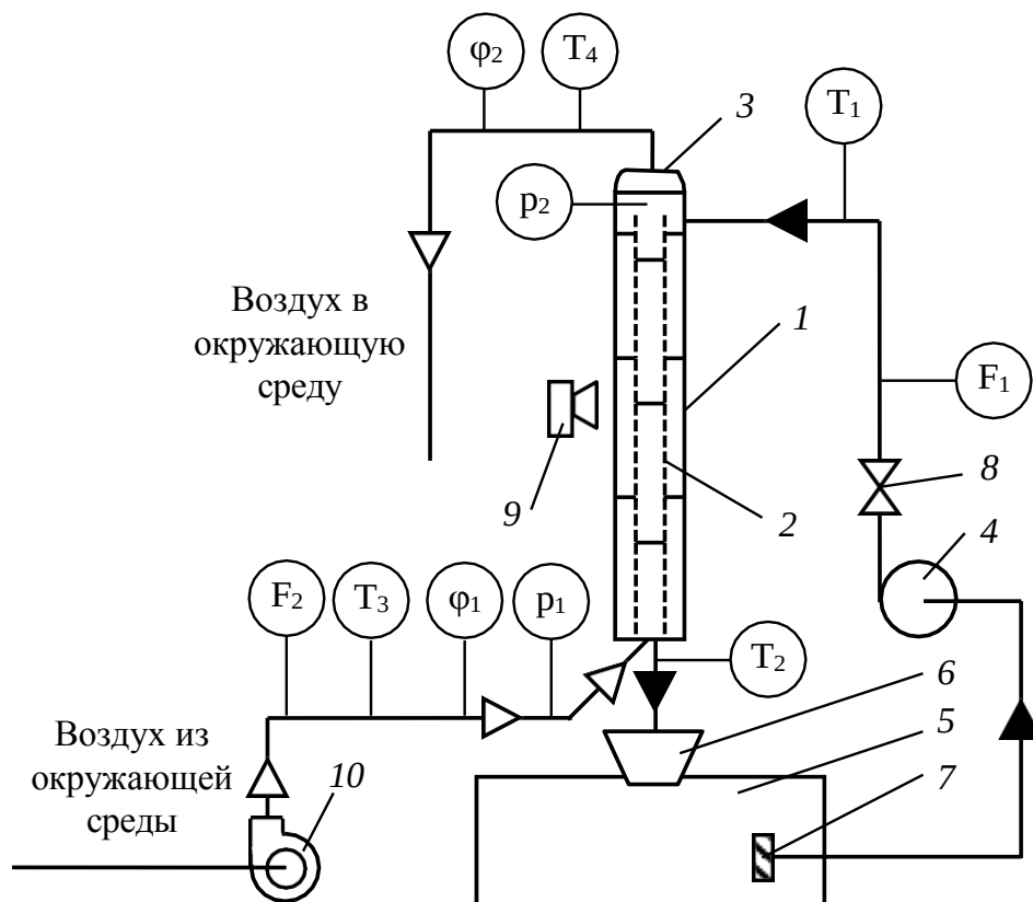
Рис. 2. Схема экспериментальной установки с вихревыми контактными ступенями:
