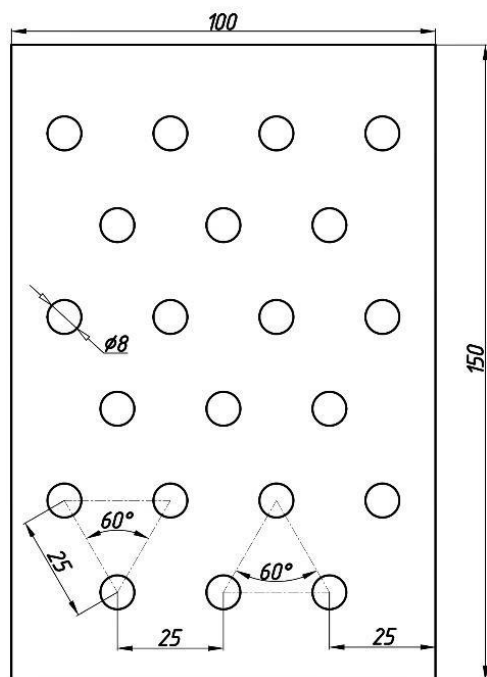
Рис. 1. Схема размещения труб в блоке оросителя по вершинам равностороннего треугольника
