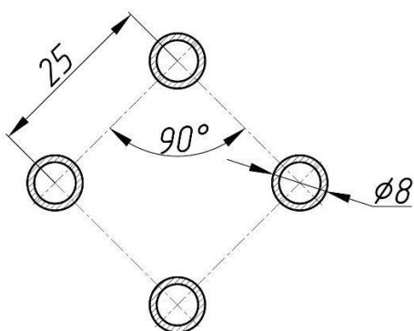
Рис. 3. Схема размещения труб по вершинам квадратов
