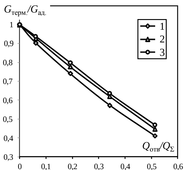
Рис. 3. Отношение массового расхода паров при термической и адиабатической ректификации в зависимости от соотношения отведенного тепла из 1-ой ступени колонны к суммарному тепловому потоку в конденсаторе и дефлегматоре при различном
