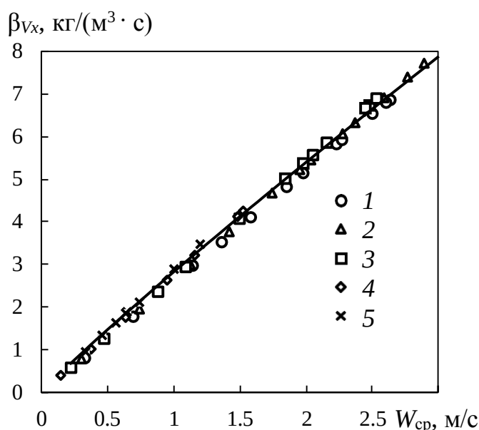
Рис. 3. Изменение объемного коэффициента массоотдачи от среднерасходной скорости воздуха при различных массовых плотностях орошения q , кг/(м 2 ·с): 1 – 4,4; 2 – 5,67; 3 – 6,63; 4 – 7,84; 5 – 12; точки – эксперимент, сплошная линия – расчет по полученному уравнению.
