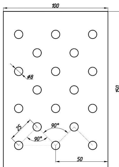
Рис. 2. Схема размещения труб в блоке оросителя по вершинам квадратов
