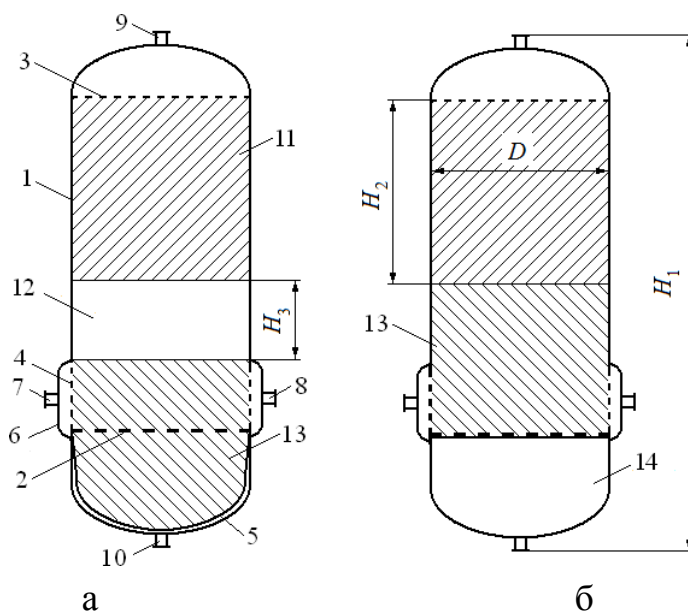
Рис. Ионообменный аппарат:
