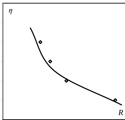
Рис. 1. Изменение среднего КПД вихревой контактной ступени в зависимости от флегмового числа при термической ректификации; сплошная линия – расчет, точки – эксперимент.
