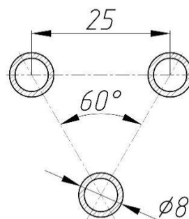
Рис. 4. Схема размещения труб по вершинам равностороннего треугольника
