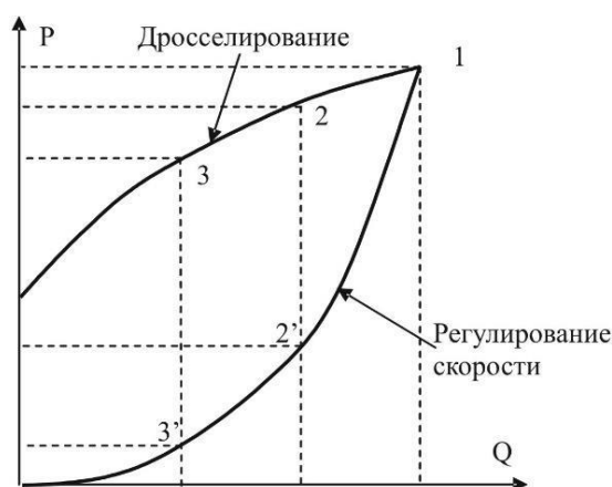
Рисунок 3. Зависимость потребляемой мощности от расхода
