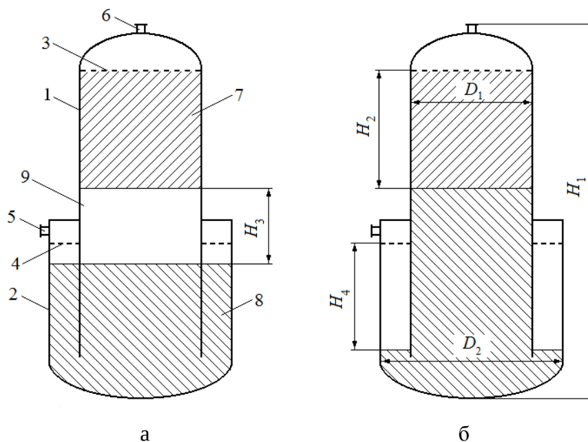
Рис. 1. Ионообменный аппарат:
