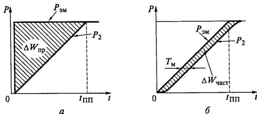
Рисунок 2. Потери энергии при прямом (а) и частотном (б) пуске
