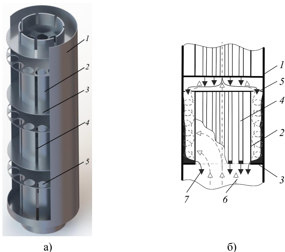
Рис. 1. 3D модель с продольным разрезом (а) и принцип работы многоступенчатой вихревой камеры (б): 1 – корпус; 2 – вихревая контактная ступень; 3 – основание; 4 – прорезы; 5 – отверстия для выхода воздуха; 6 – поток охлаждающего воздуха; 7 – поток воды.
