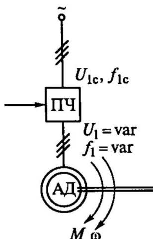
Рисунок 1. Структура частотно-регулируемого электропривода
