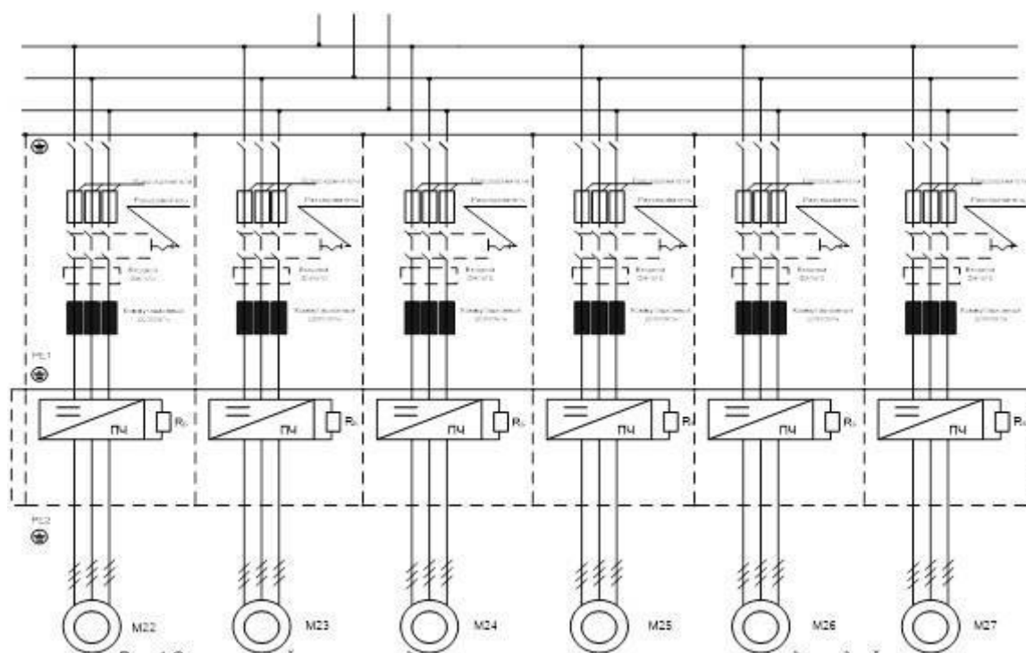
Рис.1. Схема питания многодвигательной линии обрезающего корда от индивидуальных преобразователей частоты
