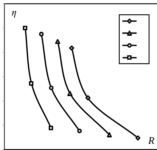
Рис. 2. Изменение среднего КПД вихревой контактной ступени в зависимости от флегмового числа при различном соотношении отведенного тепла из 1-ой ступени колонны к суммарному тепловому потоку в конденсаторе и дефлегматоре Q_{отв}/Q_{\Sigma} : 1 – 0,0616; 2 – 0,192; 3 – 0,342; 4 – 0,513.
